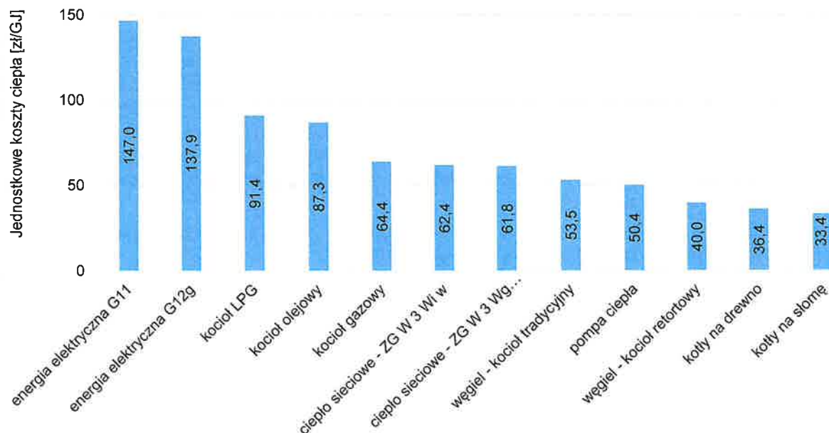
Rysunek 12 Porównanie rocznych kosztów wytworzenia energii w odniesieniu do jednostkowych wskaźników kosztów energii użytecznej dla różnych nośników Źródło: analizy własne
